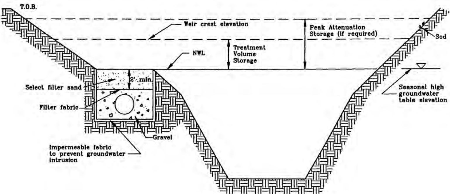
Figure 22-2. Filter shelf in a wet basin (N.T.S.)
