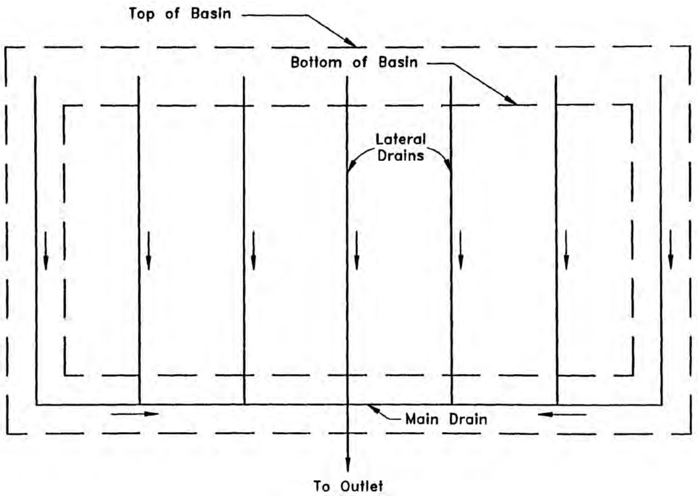
Figure 6-2. Top view of underdrain system (N.T.S.)
