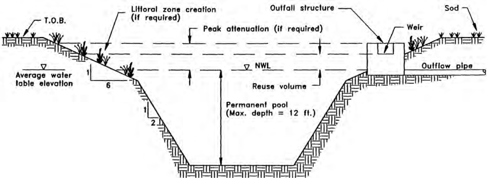
Figure 21-1. Stormwater harvesting system (N.T.S.)
