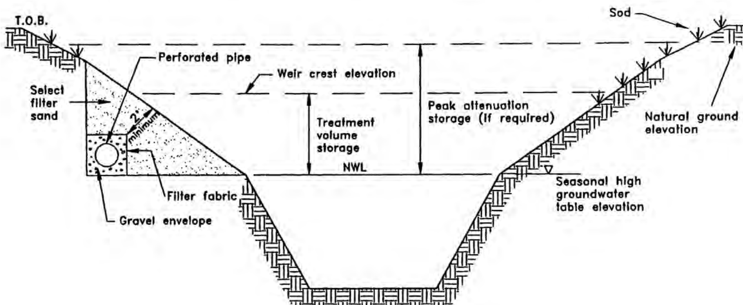
Figure 22-1. Side-bank filters in a wet basin (N.T.S.)
